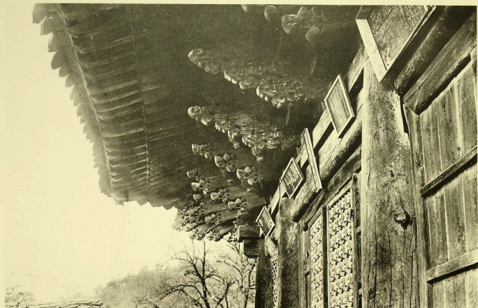
五二二 安國寺大雄殿外部正面斗拱及軒 五二三 同 寺大雄殿外部側面斗拱及軒 (平南 順川郡舍人面)
